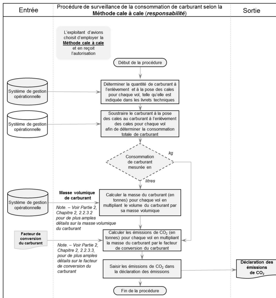
FIGURE C-5. Surveillance de la consommation de carburant par vol selon la Méthode cale à cale
