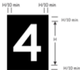
Figure A4-5. Dimensions des panneaux RDRS
