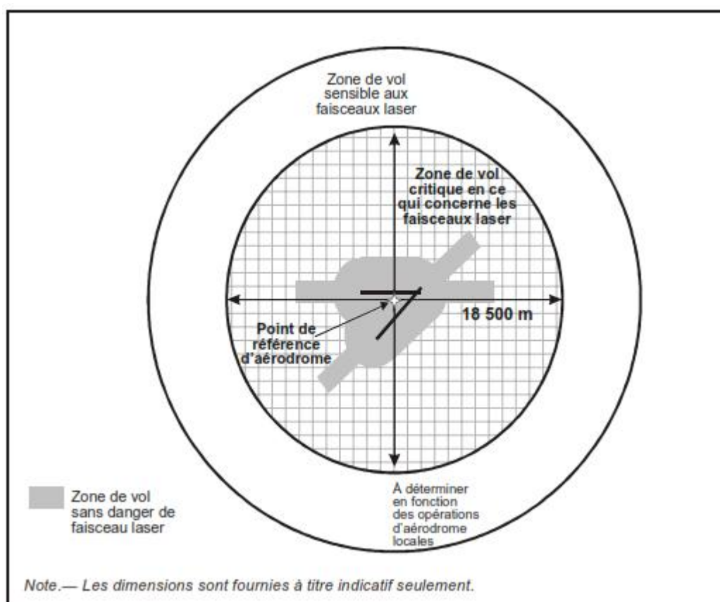
Figure5-11. Zones de vol protégées
