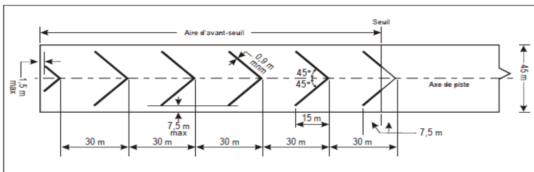
Figure 7-3. Marques d'avant-seuil
