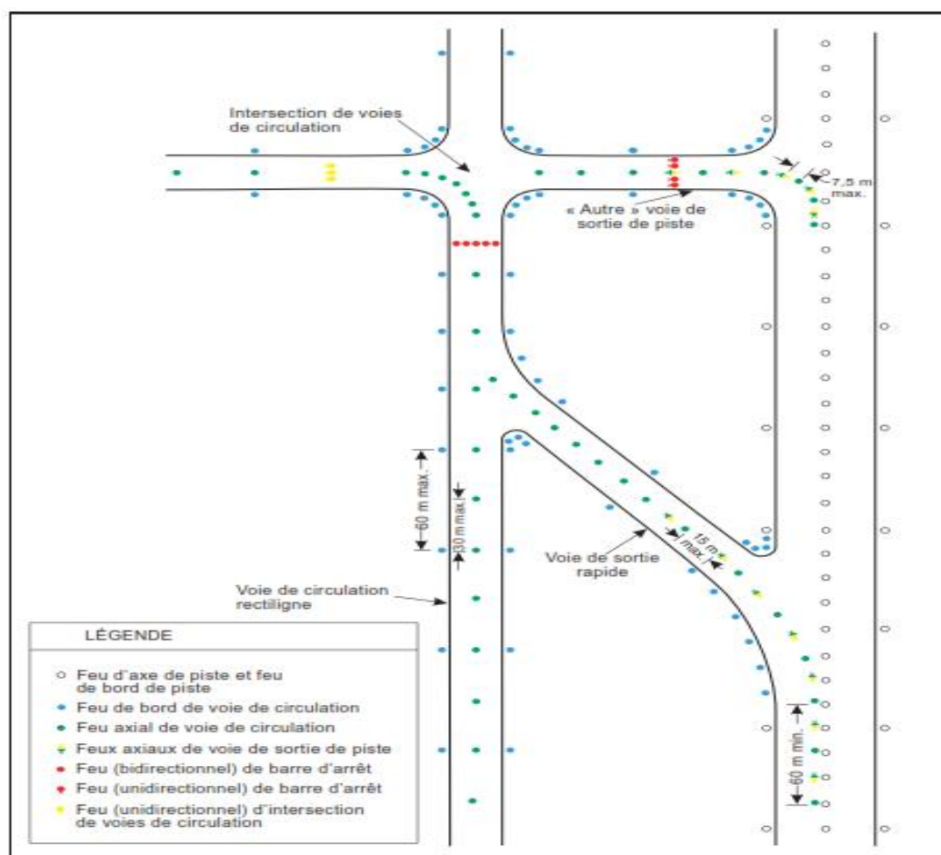
Figure 5-26 Balisage lumineux de voie de circulation
