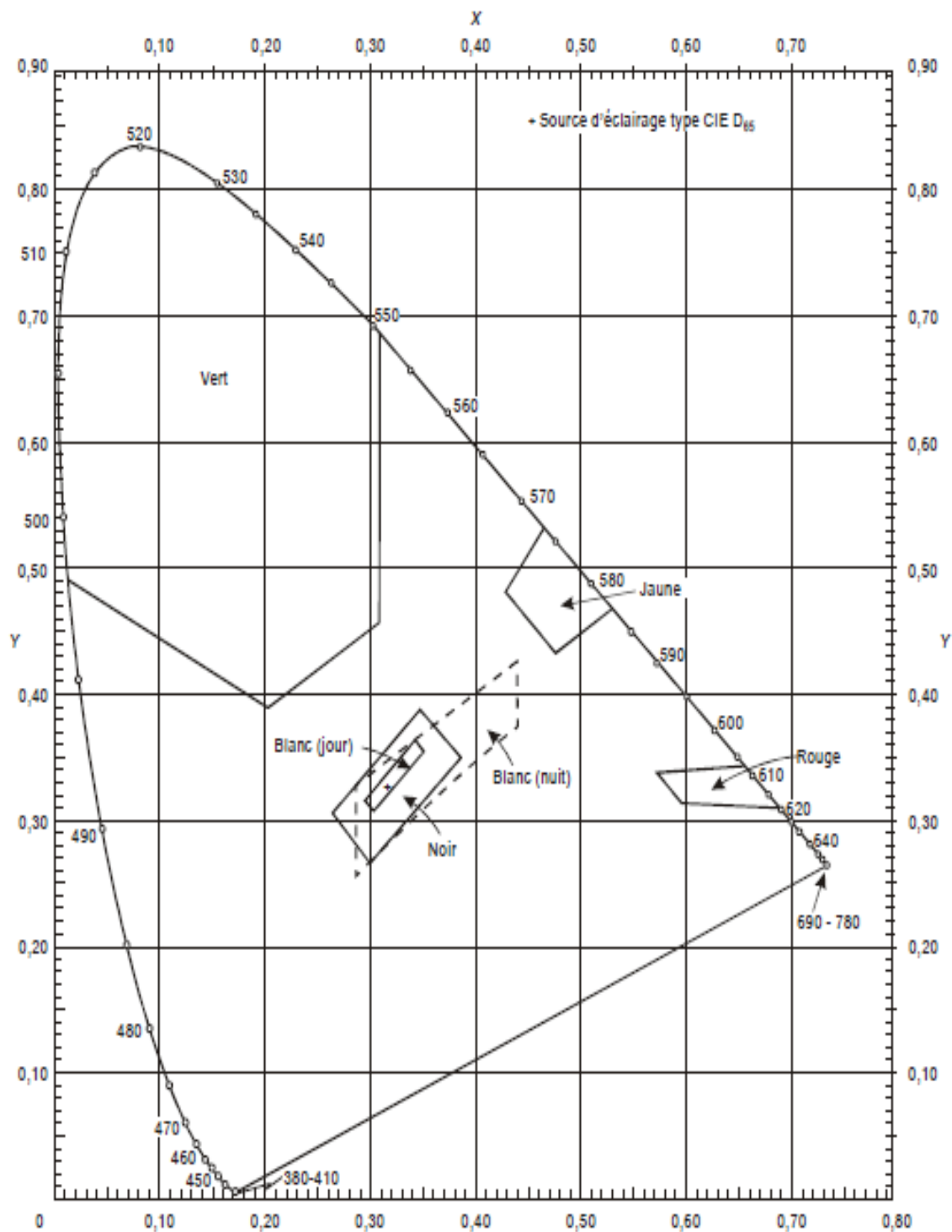
Figure A1-4. Couleurs des panneaux de signalisation et autres panneaux lumineux éclairés de l'intérieur
