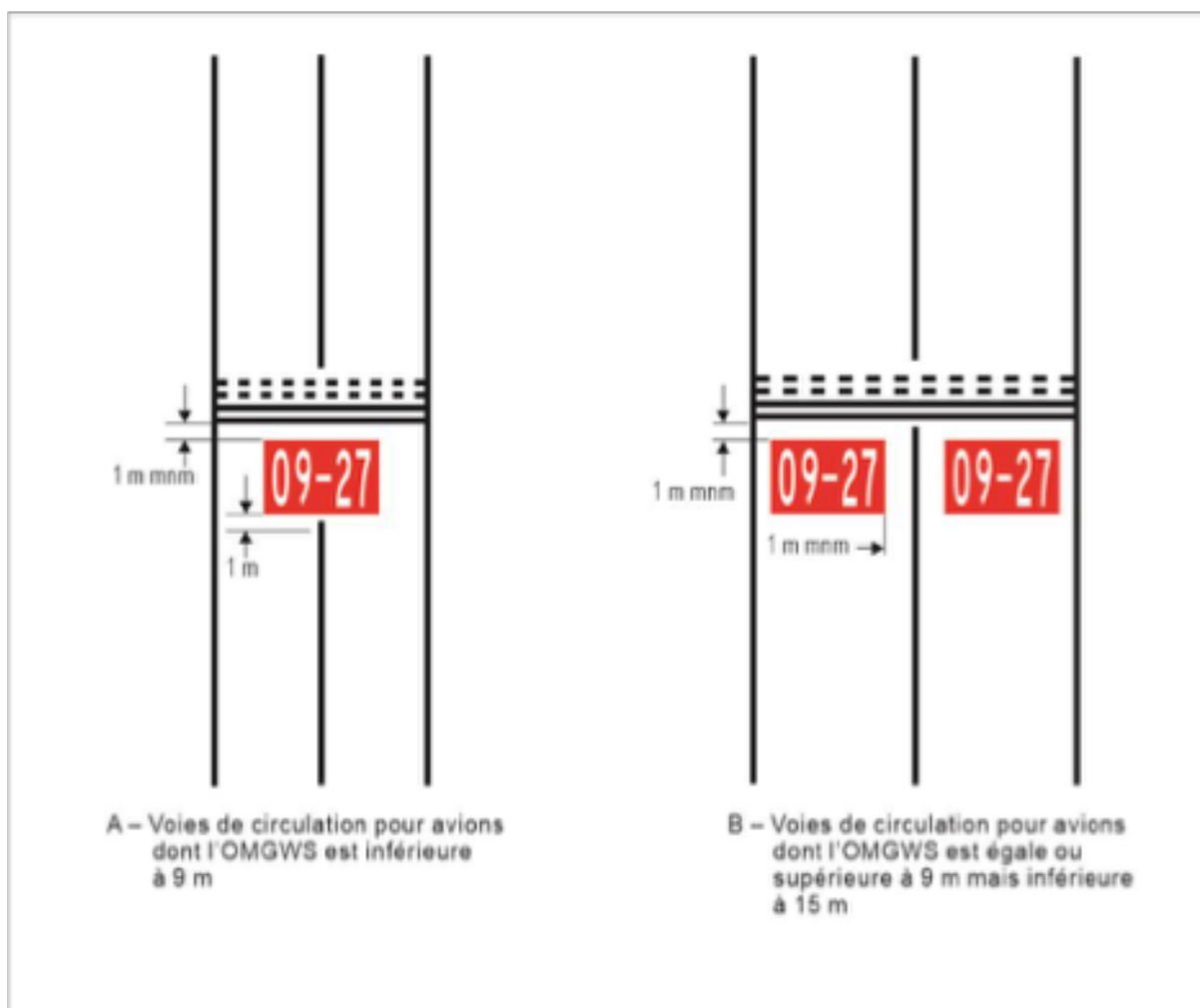
Figure 5-10. Marque d'obligation
