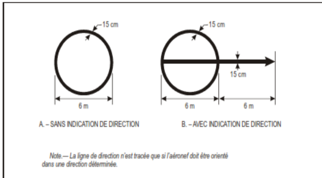
Figure 5-9. Marques de point de vérification VOR d'aérodrome
