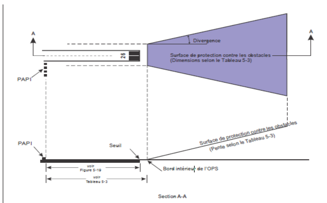
Figure 5-21. Surface de protection contre les obstacles pour les indicateurs visuels de pente
