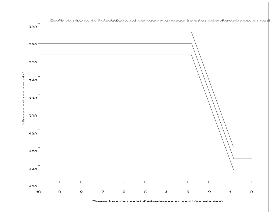
Figure D-9. Famille de profils de vitesse d'un aéronef
