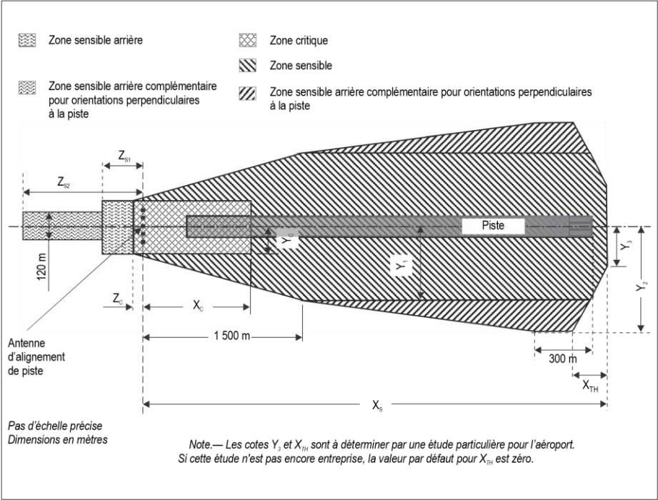
Figure C-3. Exemple de dimensionnement de la zone sensible et de la zone critique d'un radiophare d'alignement de piste (dimensions chiffrées dans le tableau C-1 qui suit)
