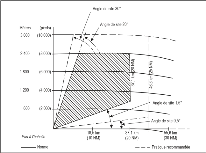
Figure C-18. Élément SRE du système radar d’approche de précision – Couverture verticale pour un aéronef de 15 m² de surface réfléchissante
