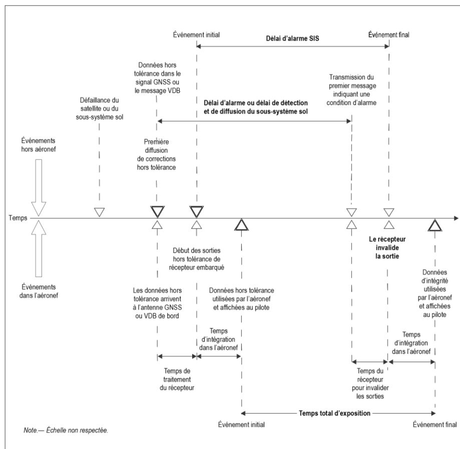
Figure D-13. Illustration du délai d'alarme nominal GBAS
