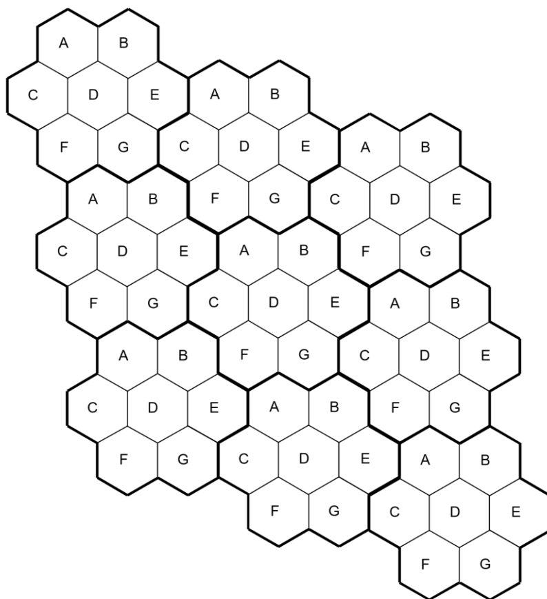
Figure D-5A. Réseau GRAS VHF à fréquence unique utilisant plusieurs créneaux temporels
