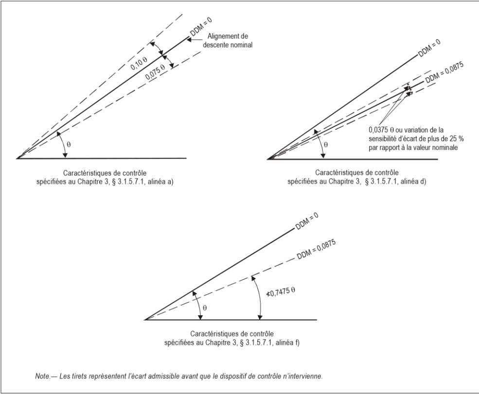
Figure C-11. Alignement de descente – Différence de modulation (DDM)
