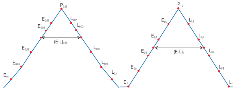
Figure D-20. Sorties de corrélateur pour les signaux Galileo E1-C ou BDS B1C_pilote (à gauche) et Galileo E5a-Q ou BDS B2a_pilote (à droite)
