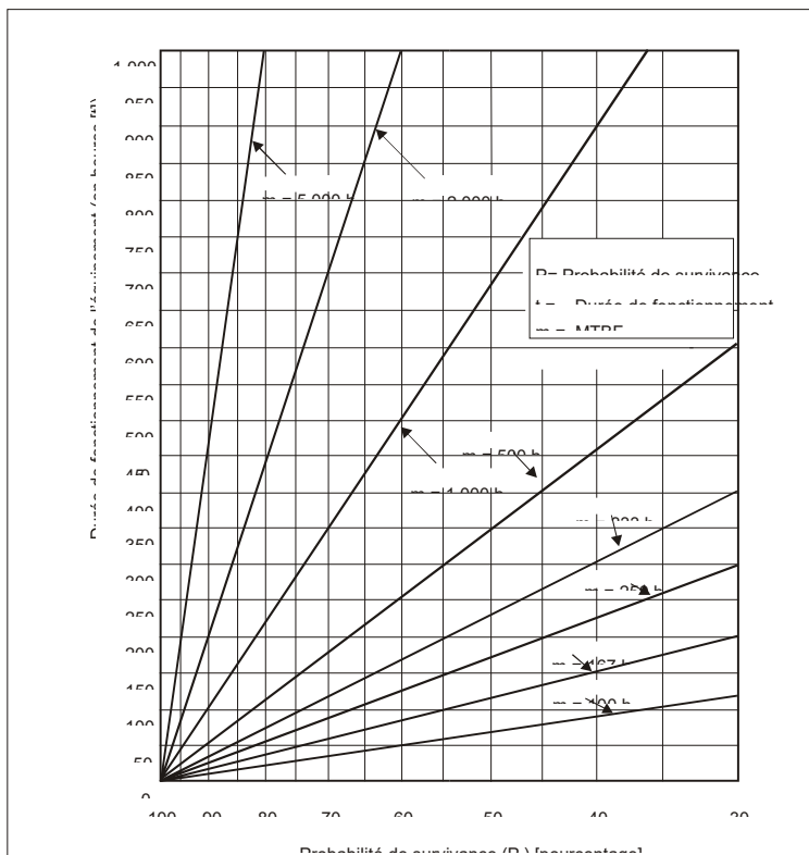
Figure F-1. Graphique de P_s = 100 e^{-t/m}
