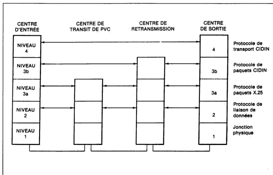
Figure 8-1. Niveaux de protocole CIDIN
