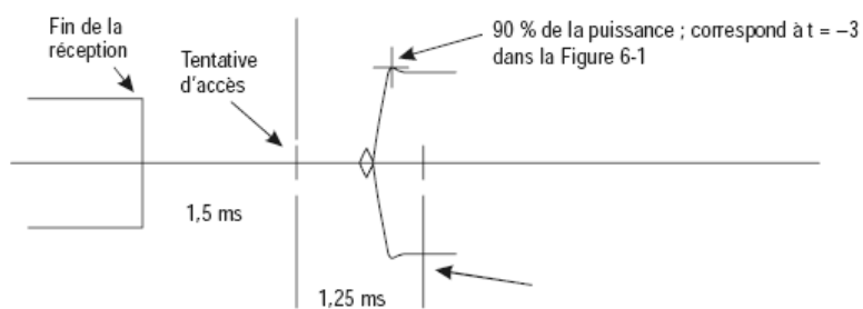
Figure 6-3. Temps de retournement réception-émission
