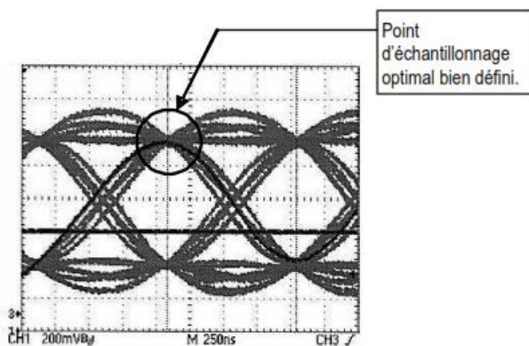
Figure 12-3. Diagramme en œil idéal
