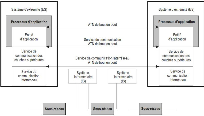
FIGURE 3-1. Modèle conceptuel de l'ATN
