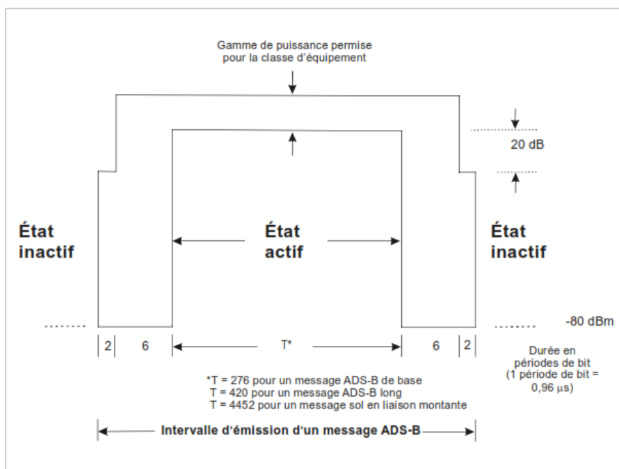
Figure 12-2. Profil temps-amplitude d'une émission d'un message UAT
