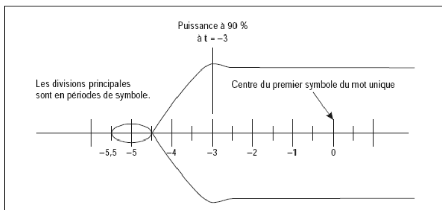
Figure 6-1. Stabilisation de la puissance de l'émetteur
