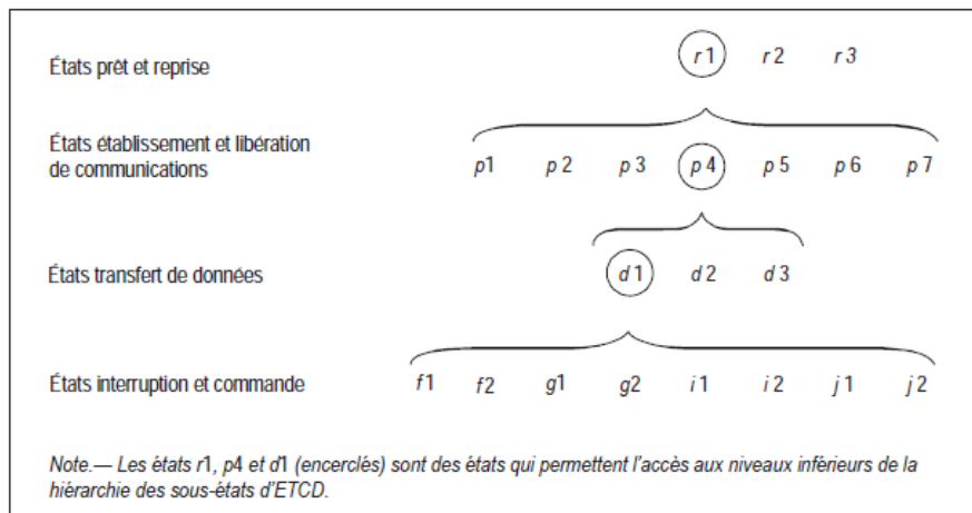
Figure 5-2. Hiérarchie des sous-états d'ETCD
