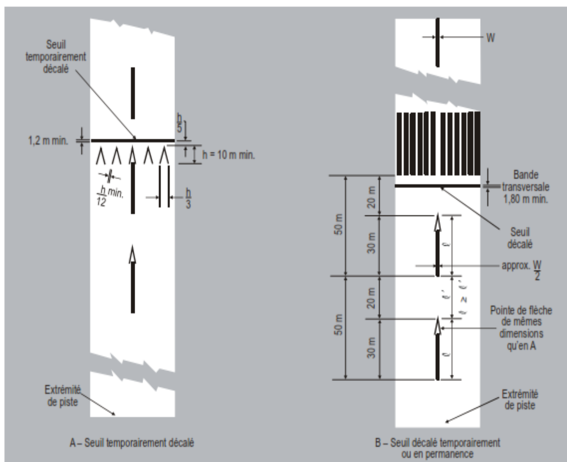
Figure 5-4. Marques de seuil décalé
