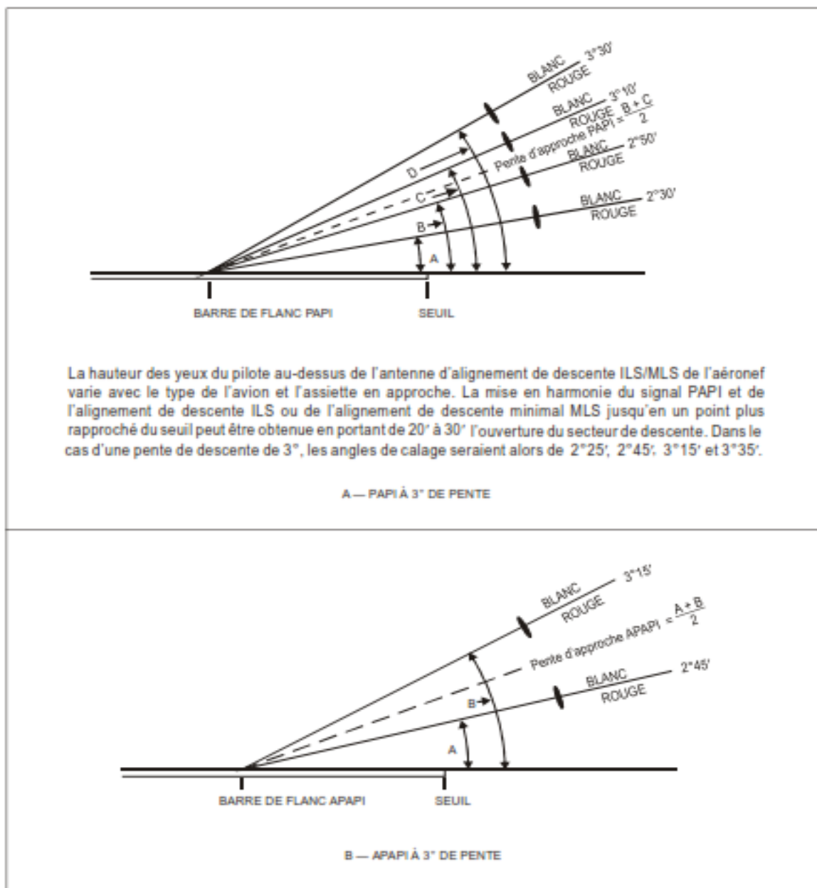
Figure 5-20. Faisceaux lumineux et calage en site d'un PAPI et d'un APAPI
