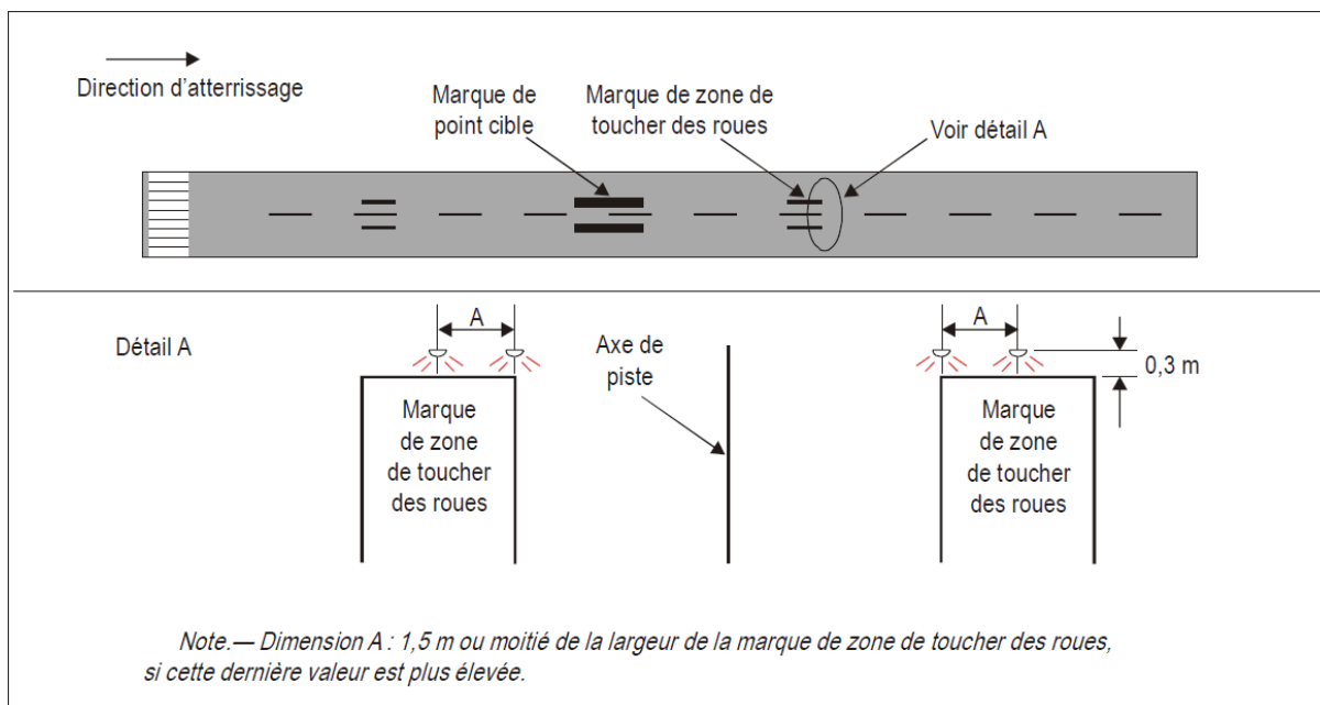
Figure 5-24. Feux simples de zones de toucher de roue
