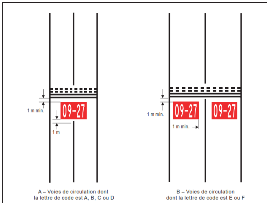
Figure 5-10. Marque d'obligation
