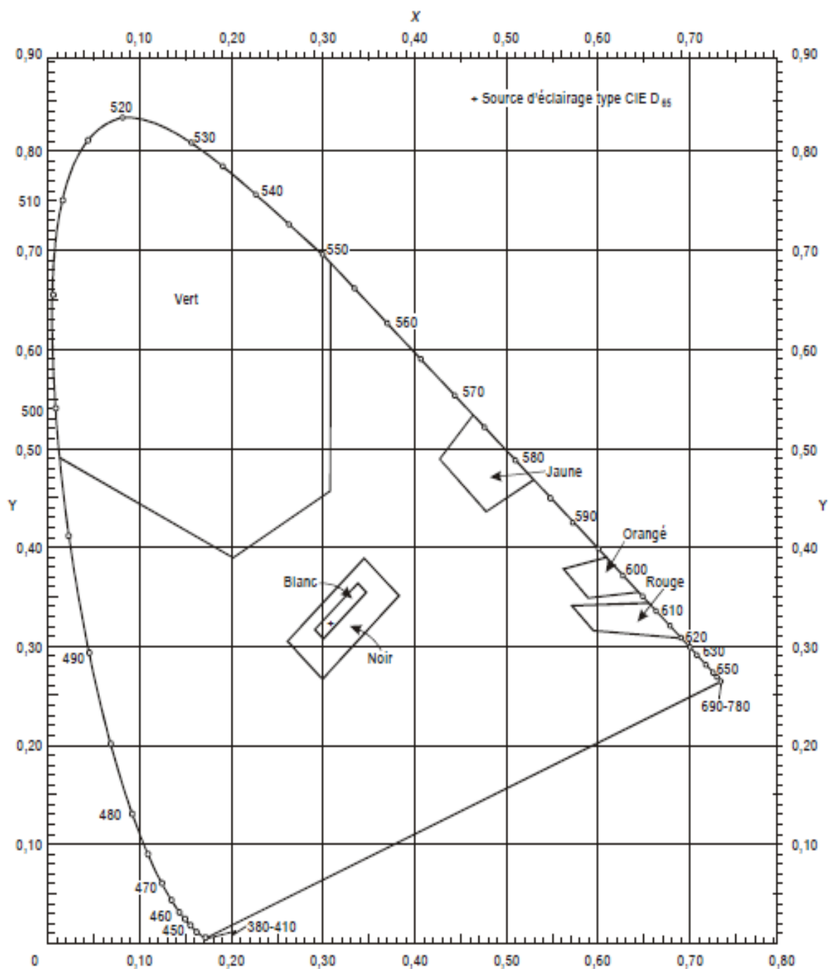
Figure A1-2. Limites recommandées des couleurs ordinaires pour les marques et les panneaux et tableaux de signalisation éclairés de l'extérieur
