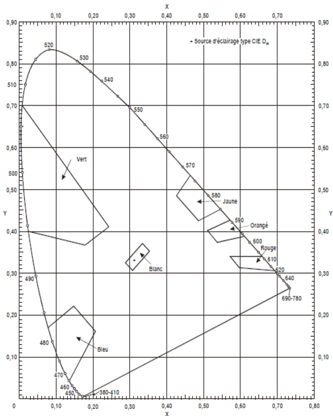
Figure A1-3. Limites recommandées des couleurs de matériaux rétro réfléchissants pour les marques et les panneaux et tableaux de signalisation
