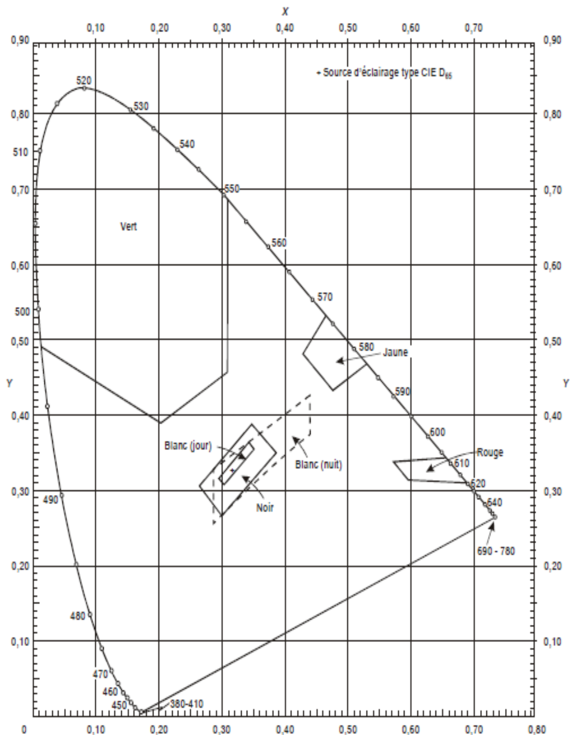
Figure A1-4. Couleurs des panneaux de signalisation et autres panneaux luminescents éclairés de l'intérieur
