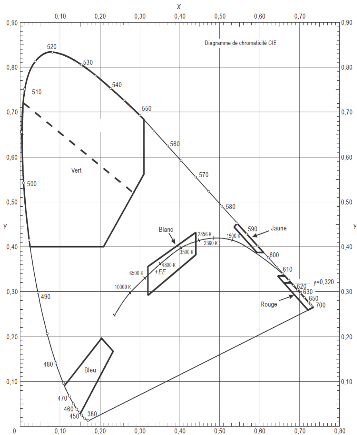
Figure A1-1b. Couleurs des feux aéronautiques à la surface (feux à semi-conducteurs)
