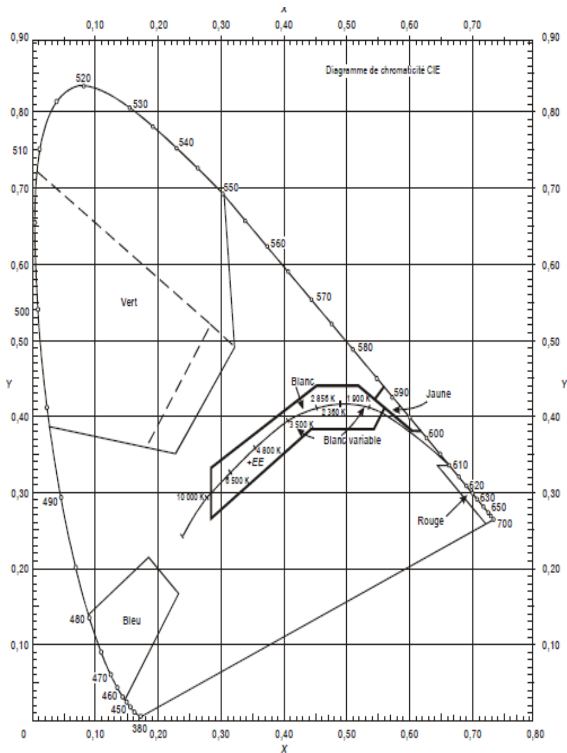
Figure A1-1a. Couleurs des feux aéronautiques à la surface (lampes à incandescence)
