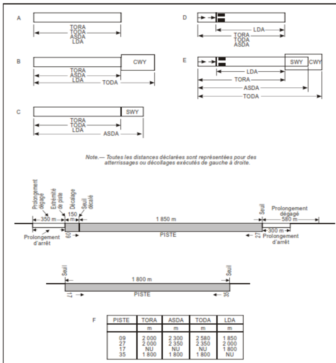
Figure A-1. Représentation des distances déclarées
