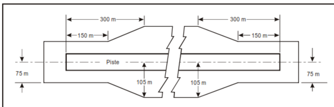
Figure A-4. Partie nivelée d'une bande de piste avec approche de précision lorsque le chiffre de code est 3 ou 4
