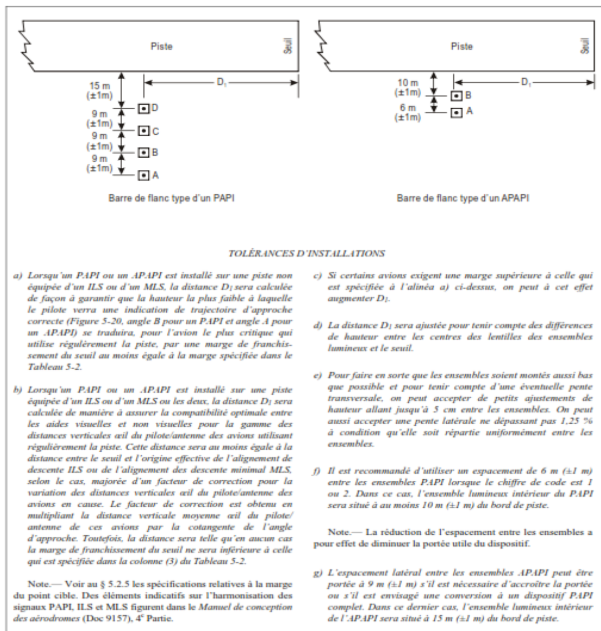
Figure 5-19. Implantation du PAPI et de l'APAPI
