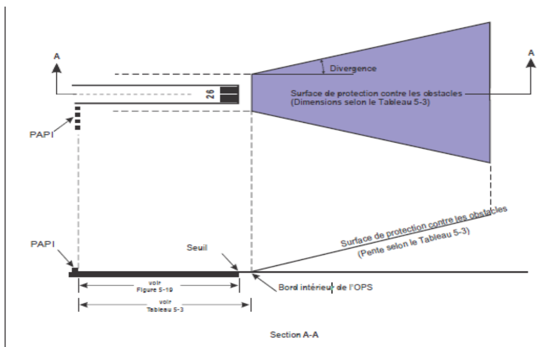
Figure 5-21. Surface de protection contre les obstacles pour les indicateurs visuels de pente d'approche
