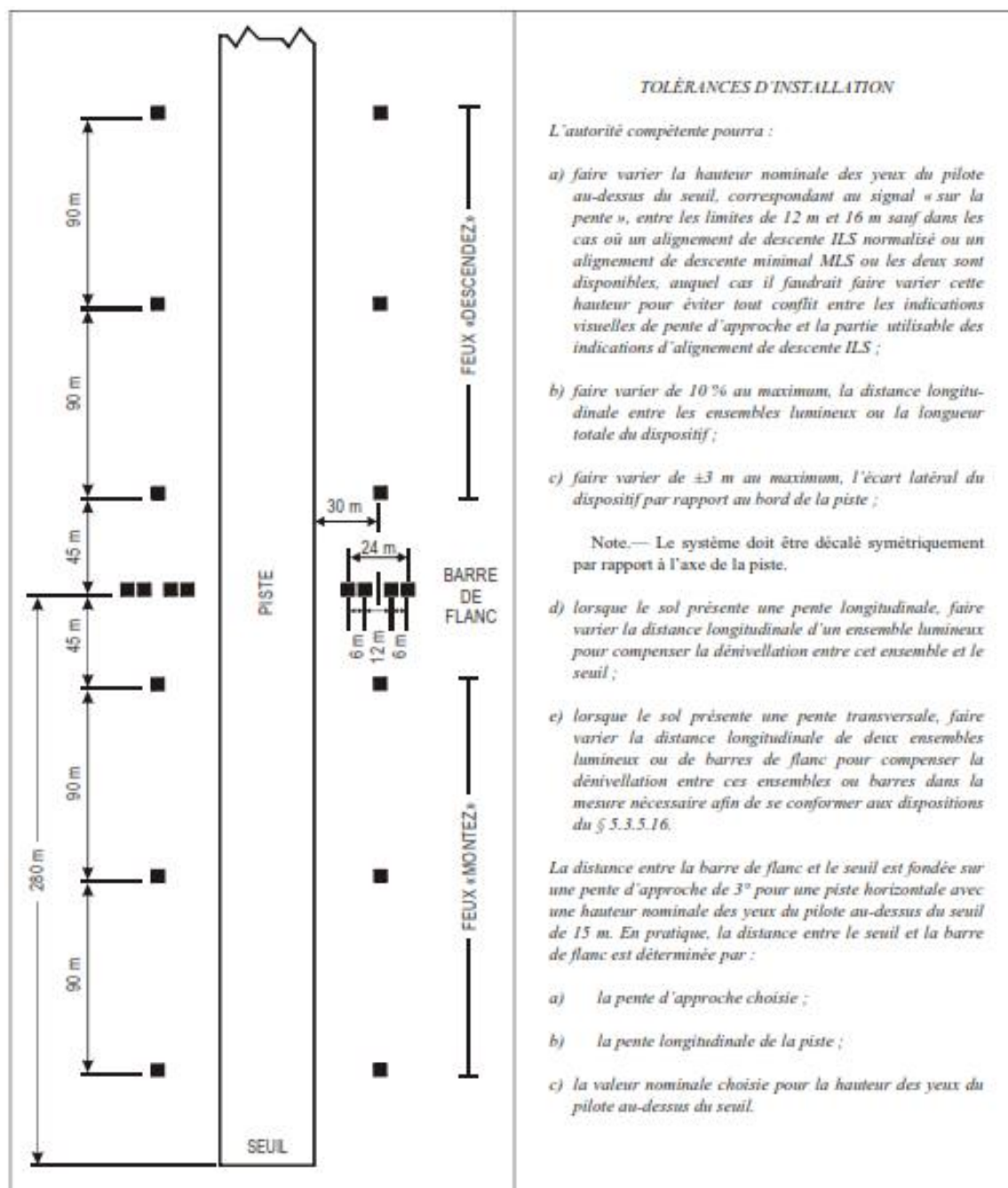
Figure 5-17. Emplacement des ensembles lumineux du T-VASIS
