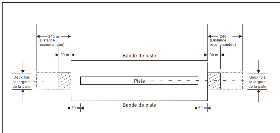
Figure A-5. Aire de sécurité d'extrémité de piste lorsque le chiffre de code est 3 ou 4
