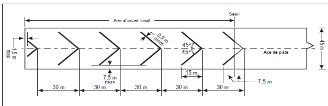
Figure 7-2. Marques d'avant-seuil
