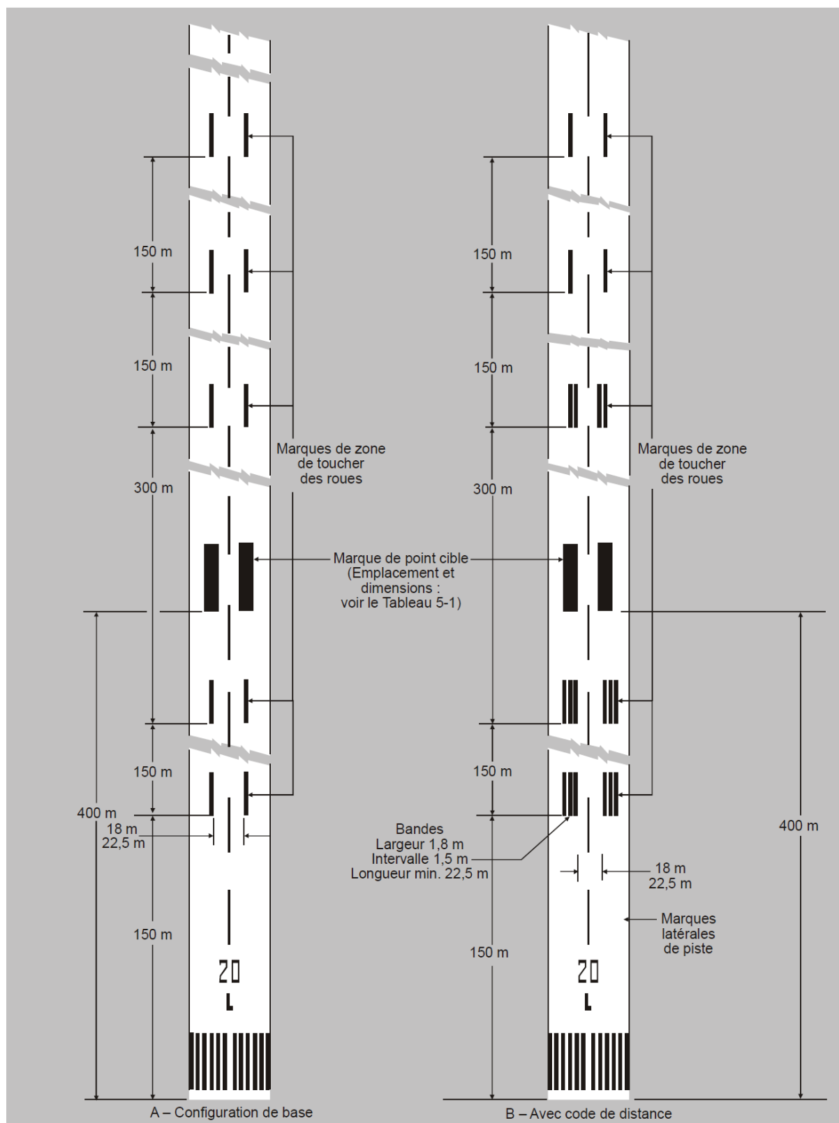
Figure 5-5. Marques de point cible et de zone de toucher des roues (la figure montre le cas d'une piste dont
