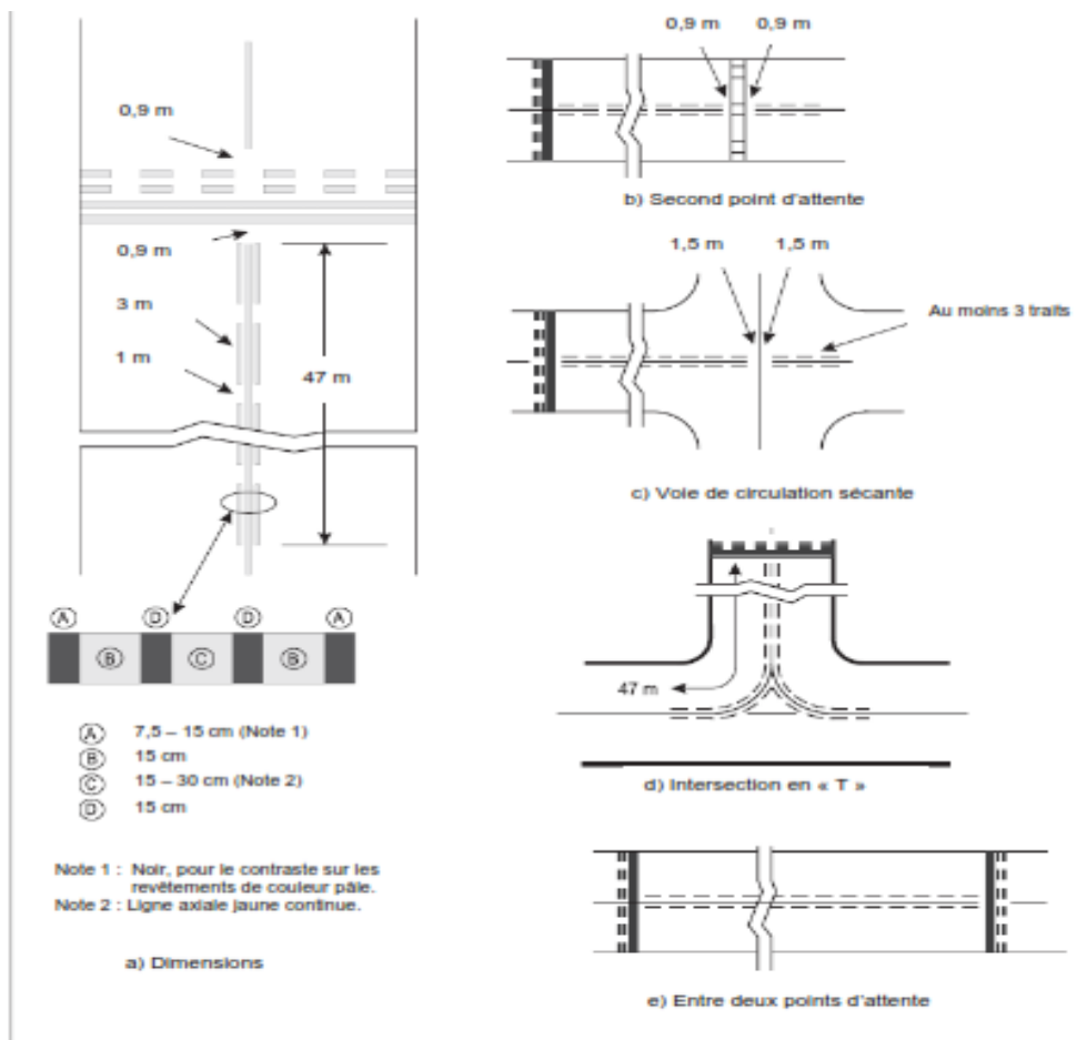
Figure 5-6. Marques de voie de circulation (représentées en association avec les marques fondamentales de piste)
