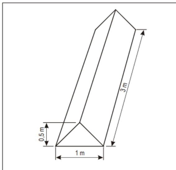
Figure 5-34. Balise de délimitation
