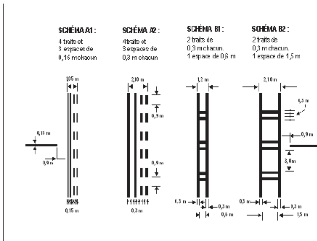
Figure 5-8. Marques de point d'attente avant piste
