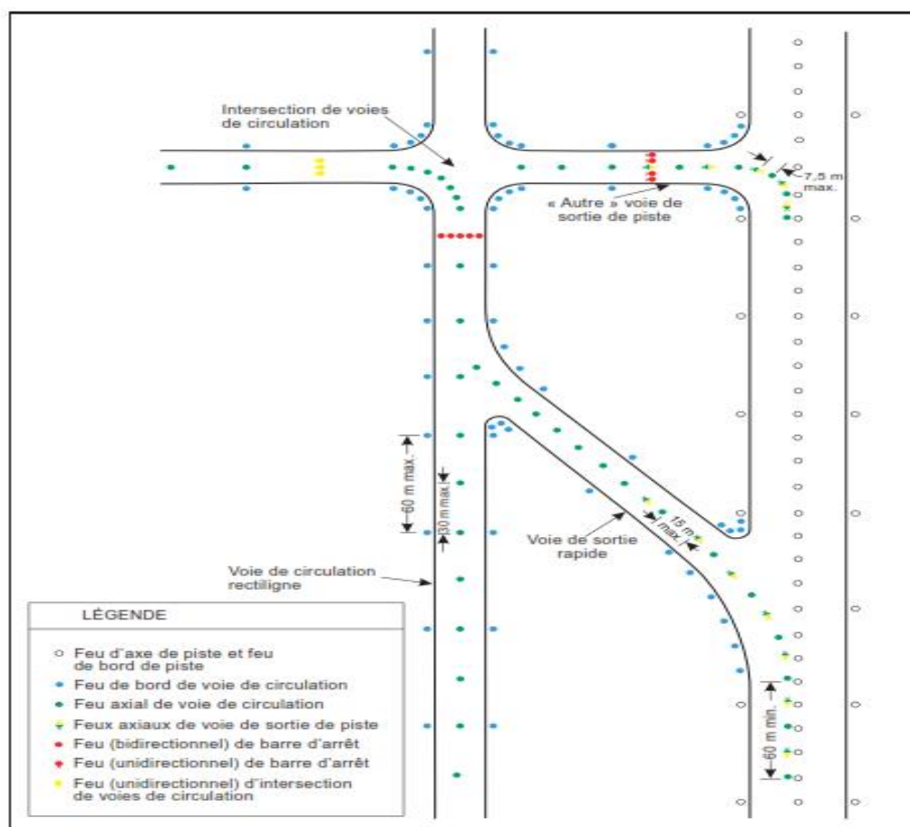
Figure 5-26 Balisage lumineux de voie de circulation
