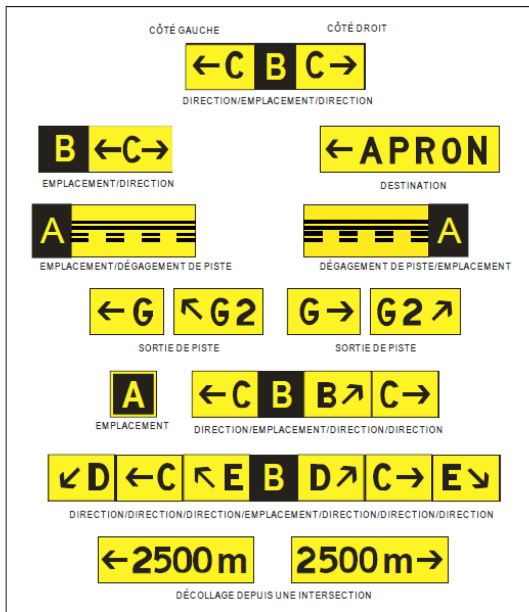
Figure 5-31 Panneaux d'indication
