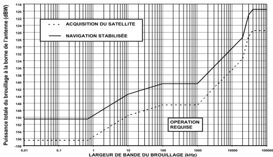
Figure B-17. Seuil de brouillage en fonction de la largeur de bande des récepteurs GPS et SBAS
