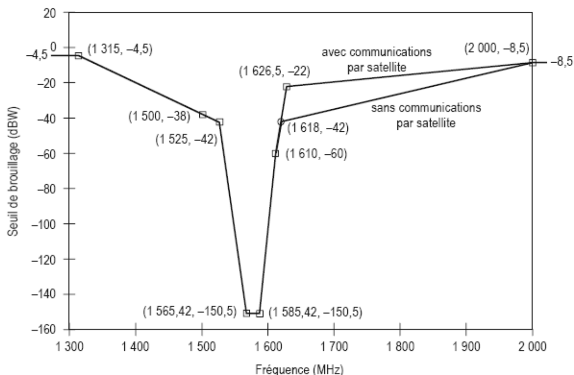
Figure B-15. Brouillage par ondes entretenues : seuils de brouillage des récepteurs GPS et SBAS en mode de navigation stabilisée
