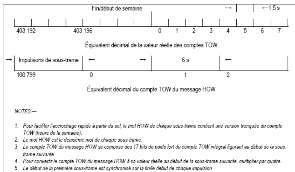
Figure B-5. Schéma temporel du HOW
